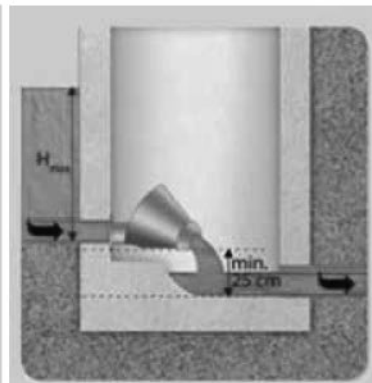
Rys. 6 Regulator stożkowy (CYDK, CYDV, CYDX) instalowany na półsucho
