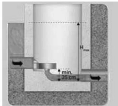
Rys. 7 Regulator poziomy (CEH) instalowany na półsucho
