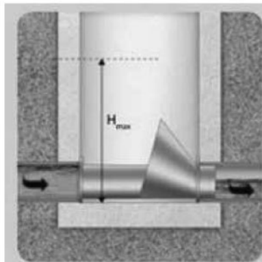
Rys. 5 Regulator stożkowy (CYDK, CYDV, CYDX) instalowany na sucho
